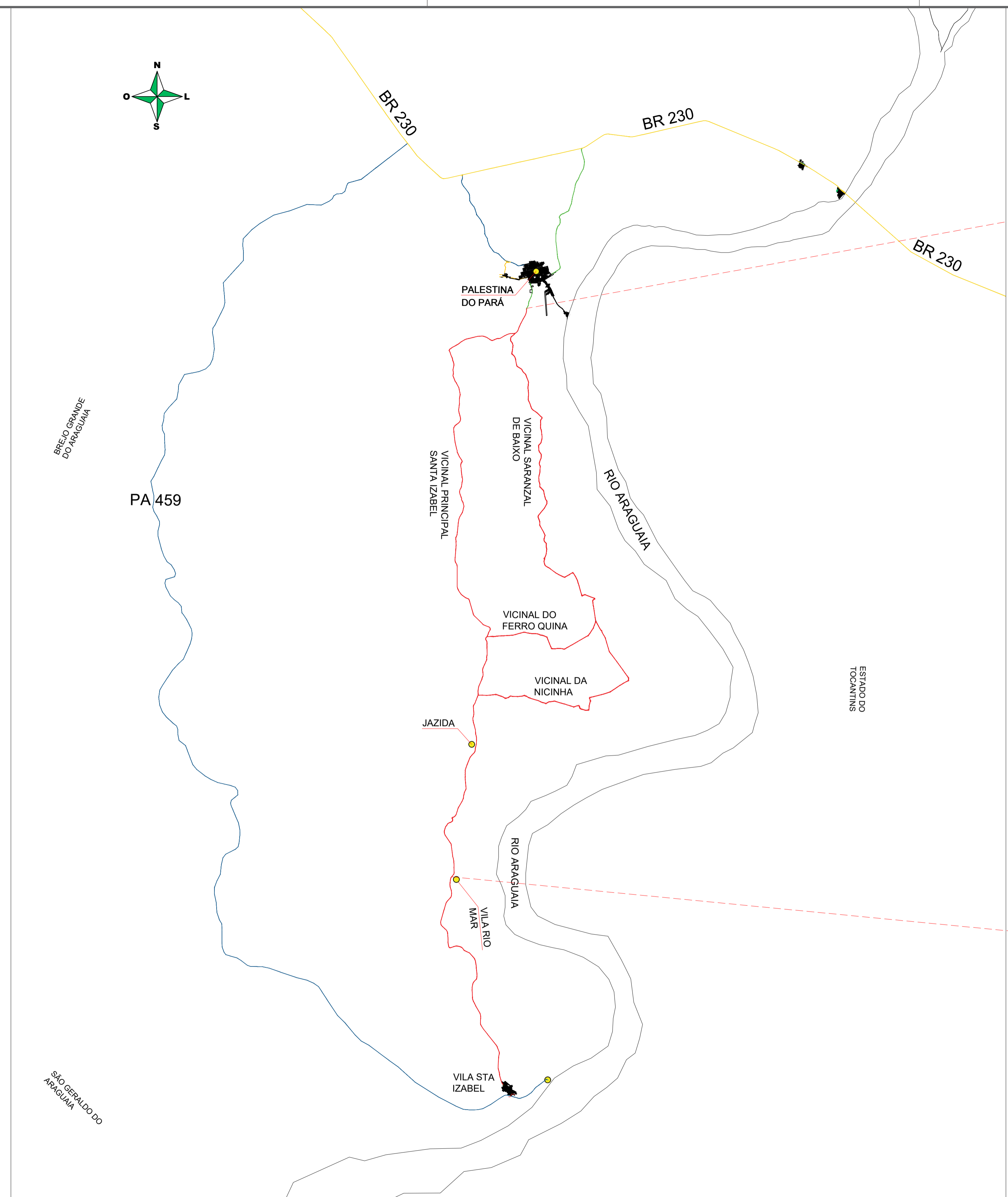
02 LOCALIZAÇÃO DO VICINAL ESCALA 1 / 1.200
